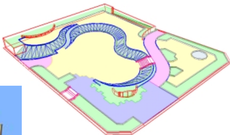
CADによる3次元作図
