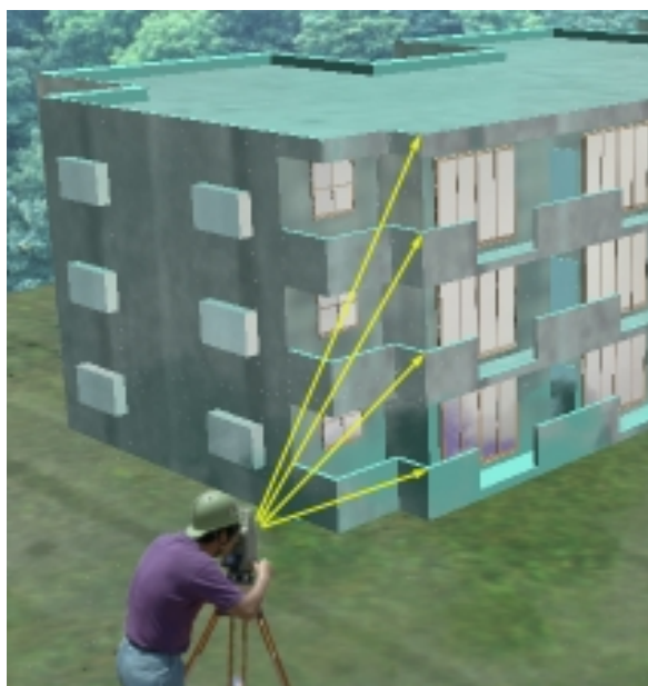
ライカによる壁面測定
